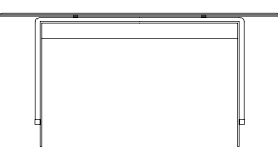
GLA.541.A L 190 D 46 H 90 cm
