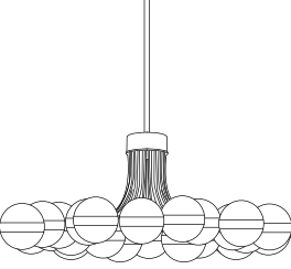
MOL.615.B 24-light chandelier Ø 180 H 70 cm
