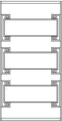
DAL.241.A L 120 D 40 H 230 cm
